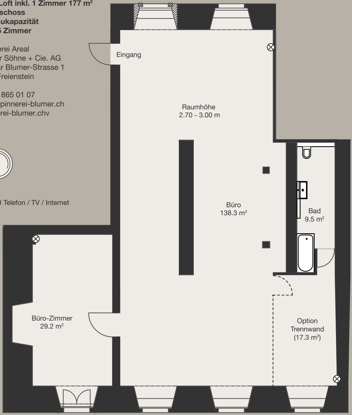
Grundriss 1. Obergeschoss
