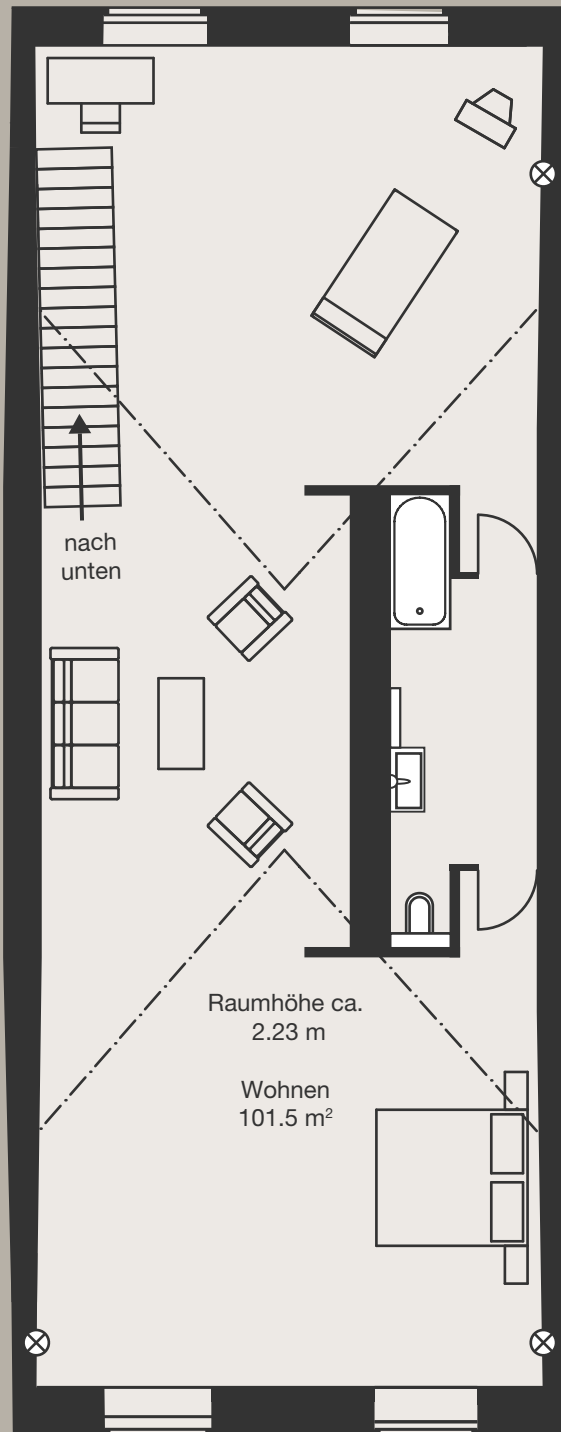
Grundriss 1. Dachgeschoss
