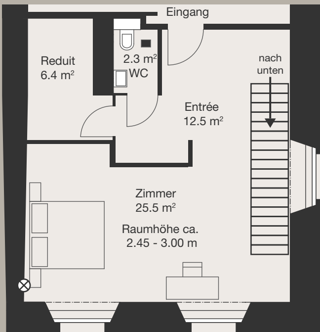
Grundriss 4. Obergeschoss
