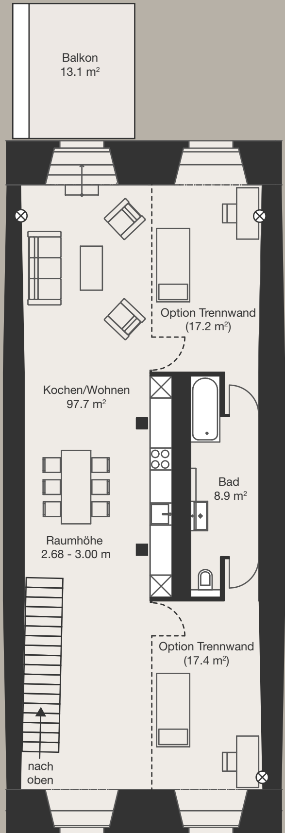
Grundriss Erdgeschoss
