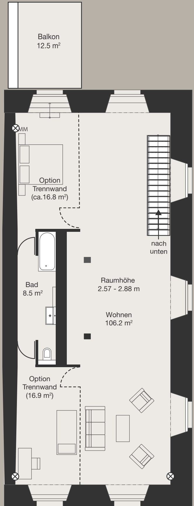
Grundriss 2. Obergeschoss
